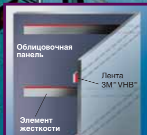
Дирборн Центр, Чикаго, Иллинойс, США. Застройщик: «Копер-Сэйлз Уна-Клад», 2003. Элементы жесткости приклеены к наружным металлическим облицовочным панелям
