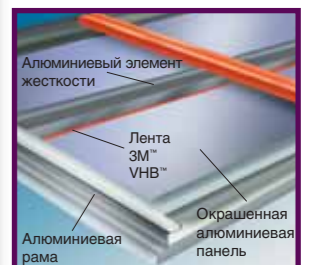
Медицинский центр Самсунг, Сеул, Южная Корея. Архитектор: «Саму Аркитектс энд Инжинирз», 1995. Алюминиевые элементы жесткости приклеены к алюминиевым панелям
