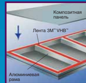
Отель «Бурж Аль Араб», Дубай, ОАЭ. Архитектор: «У. С. Аткинс и партнеры», 1999. Алюминиевые композитные панели приклеены к рамам для противодействия высоким ветровым нагрузкам
