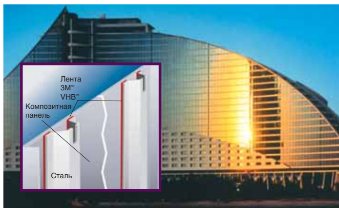
Отель «Джумейра Бич», Дубай, ОАЭ. Дизайн фасада: Schmidlin AG, 1998. Алюминиевые панели приклеены на стальные ребра жесткости
