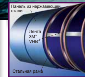
Аэропорт Форталеза, Форталеза, Бразилия. Архитектор: Клаудио Сильва, 1977. Панели из нержавеющей стали приклеены к стальной раме
